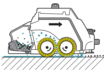
Schematische Darstellung eines Walzenbürstenkopfes mit Vorkehrfunktion
